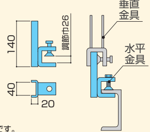
水平金具
