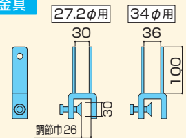
水平金具
