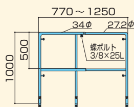
ステップスルー4型
