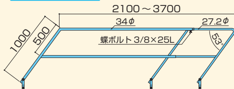
ステップスルー1型
