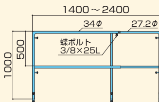
ステップスルー3型
