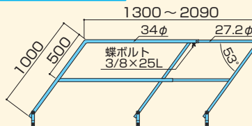
ステップスルー2型
