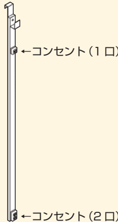
【電材モール B】 ㊦ W60×H2,082×D106 (2.9kg)
