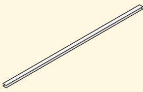
【Hジョイナー】 W50×H2,200×D32 (1.0kg)
