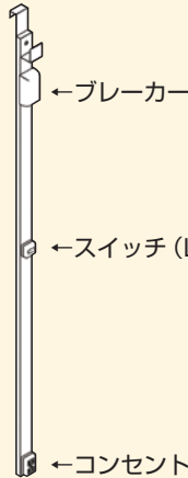
【電材モール A】 ㊦ W60×H2,082×D106 (2.9kg)
