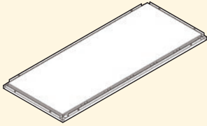
【床フレーム】 W2,180×H71.5×D900 (35.7kg)
