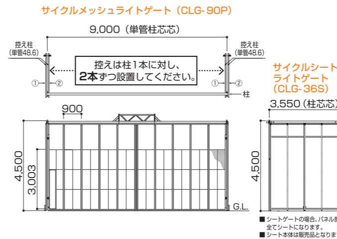
サイクルメッシュライトゲート/サイクルライトゲート/サイクルシートライトゲート H=4,500mm
